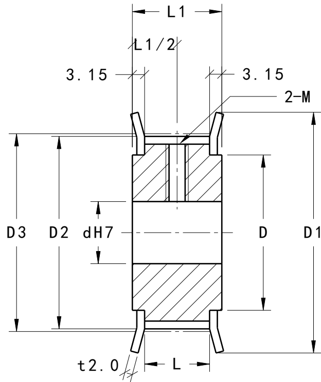
剖面視圖A-A 縮放: 1:1
