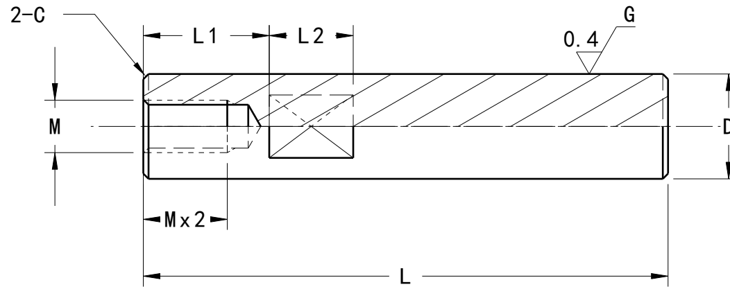
Section view A-A Scale: 2:1
