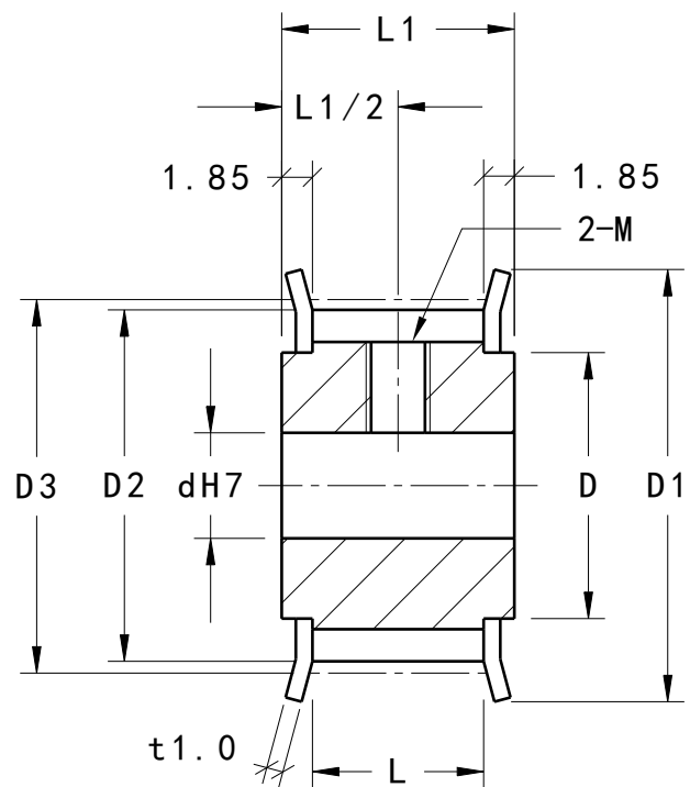
剖面視圖A-A 縮放: 2:1
