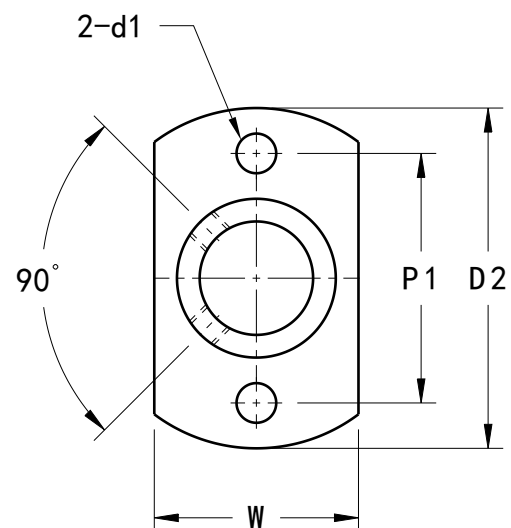
Front view[2] Scale: 3:2
